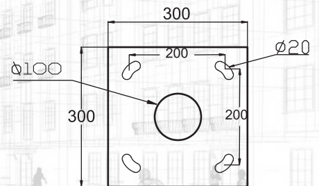
Platine d'ancrage
